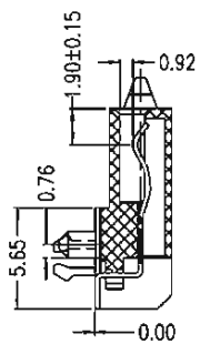
SECT A-A
