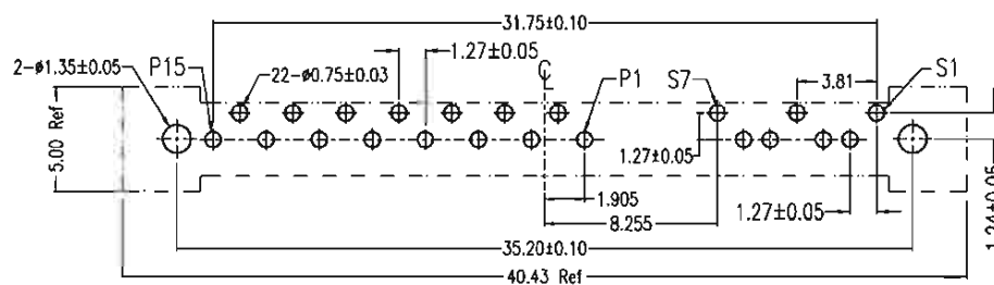
PCB Layout(T=1.6±0.05mm) TOP View
