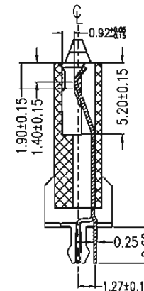
SECT A-A
