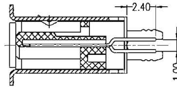
SECT A-A
